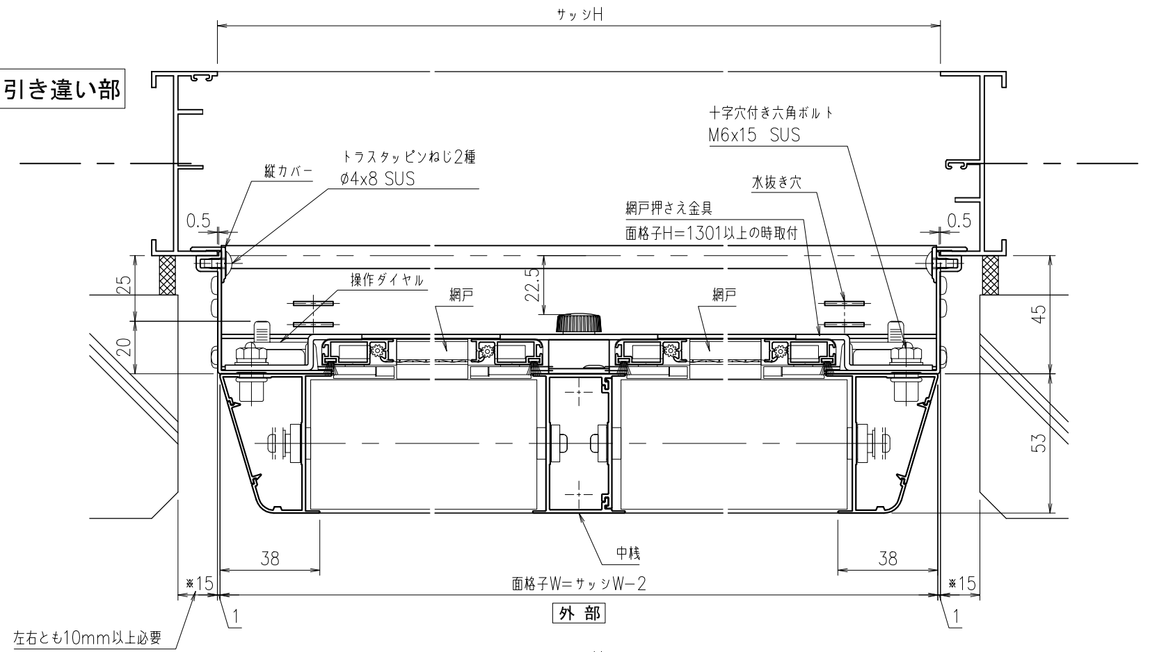
下部 FIX部
